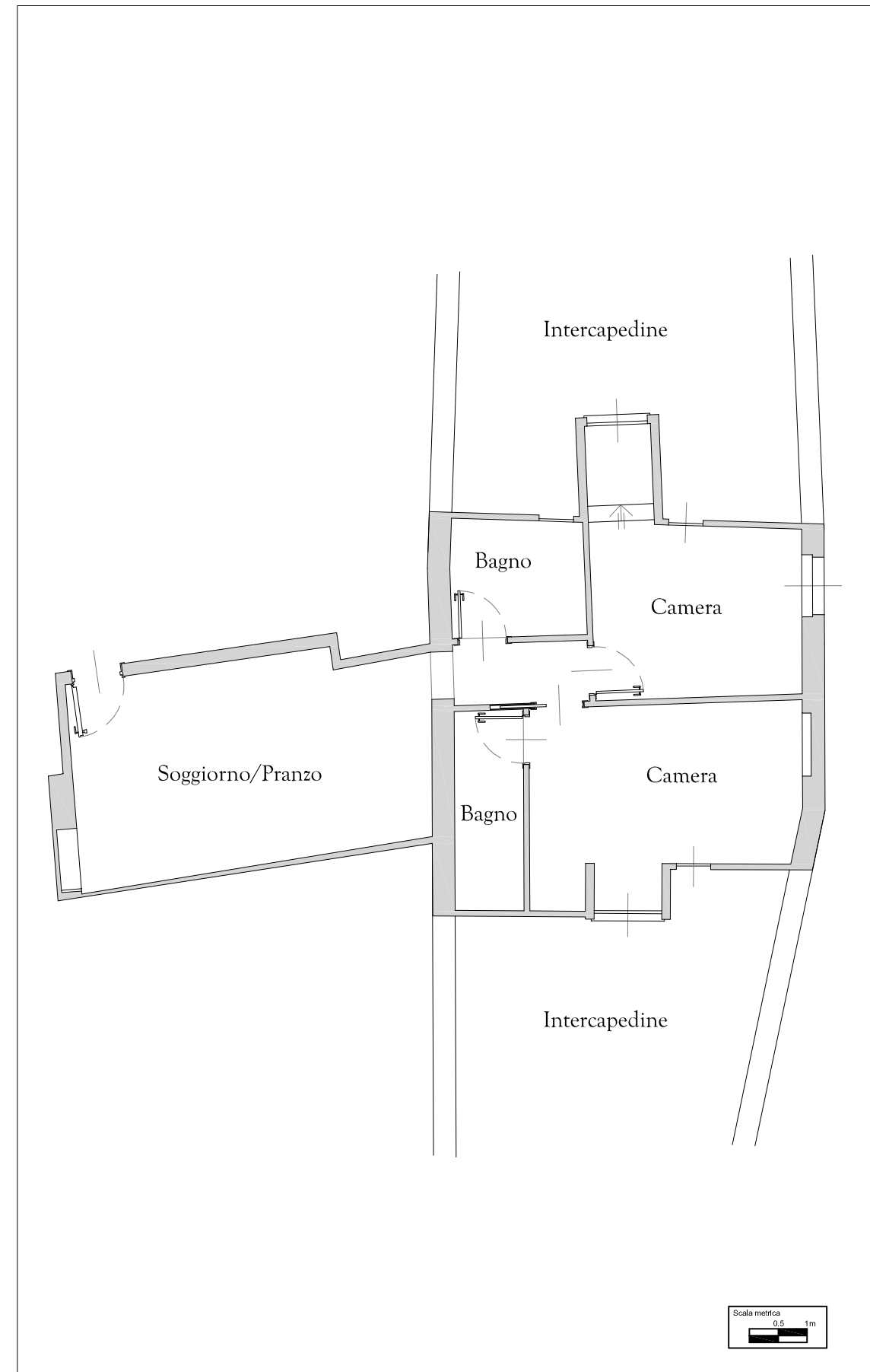
PLANIMETRIA GENERALE
